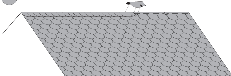
Obr. 8 - Osazení tvarovek
