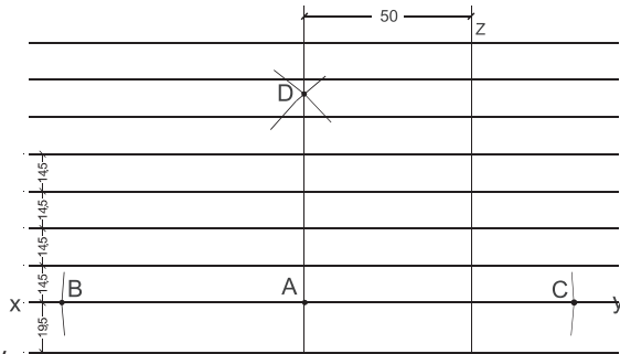
Obr. 1 - Rozvržení krytiny
