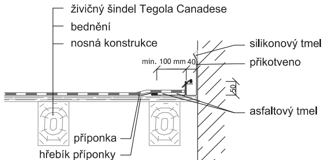
Obr. č. 12 - Napojení na svislou stěnu
