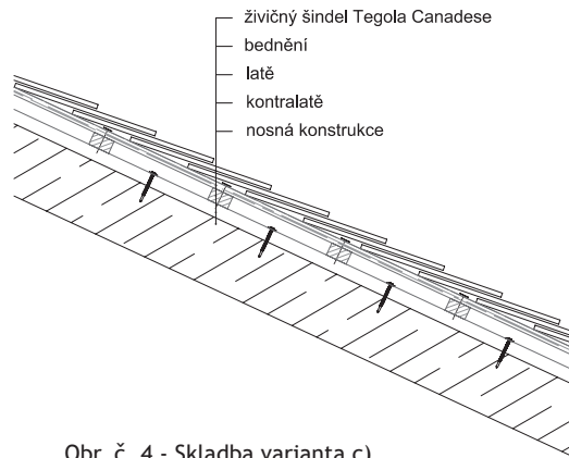
Obr. č. 4 - Skladba varianta c)
